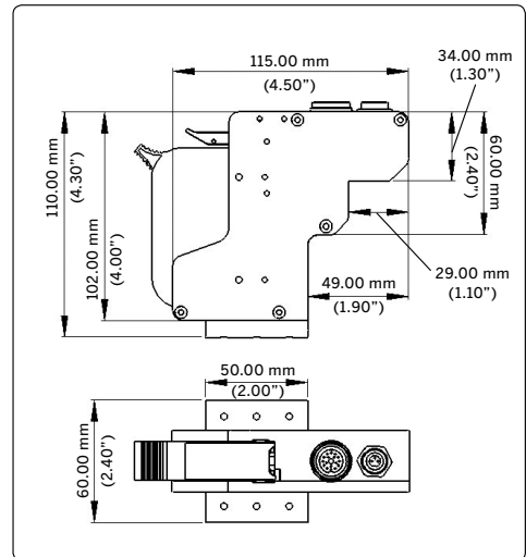
Standard Blue 프린트 헤드
